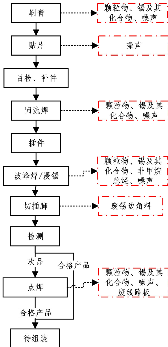
图4 本项目线路板产品生产工艺流程图
