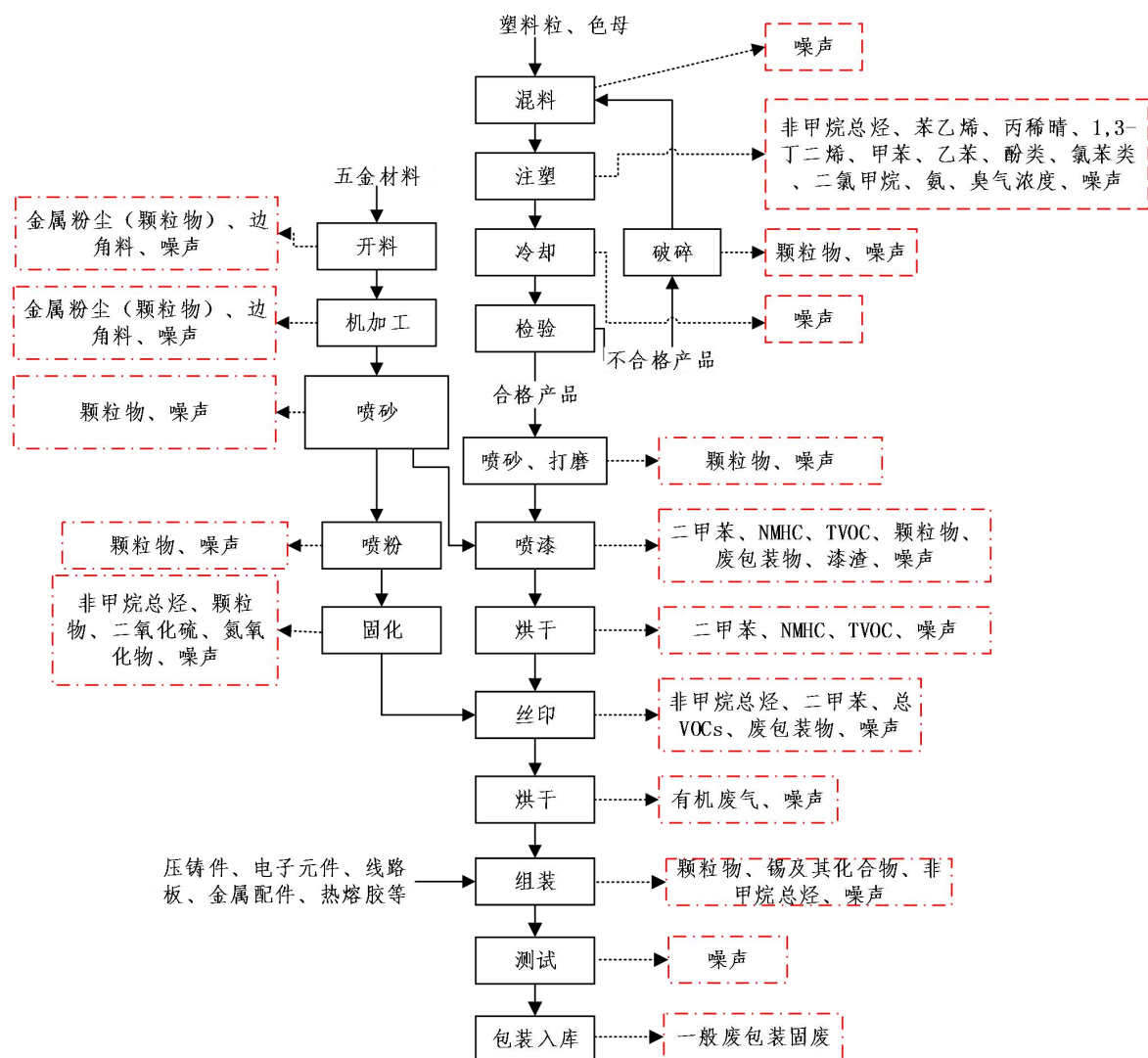
图5 项目麦克风、功放产品生产工艺流程及产污过程图
