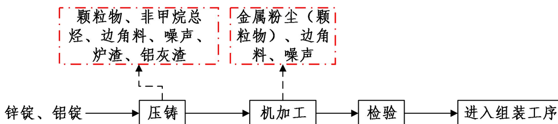
图3 项目压铸配件生产工艺流程及产污过程图
