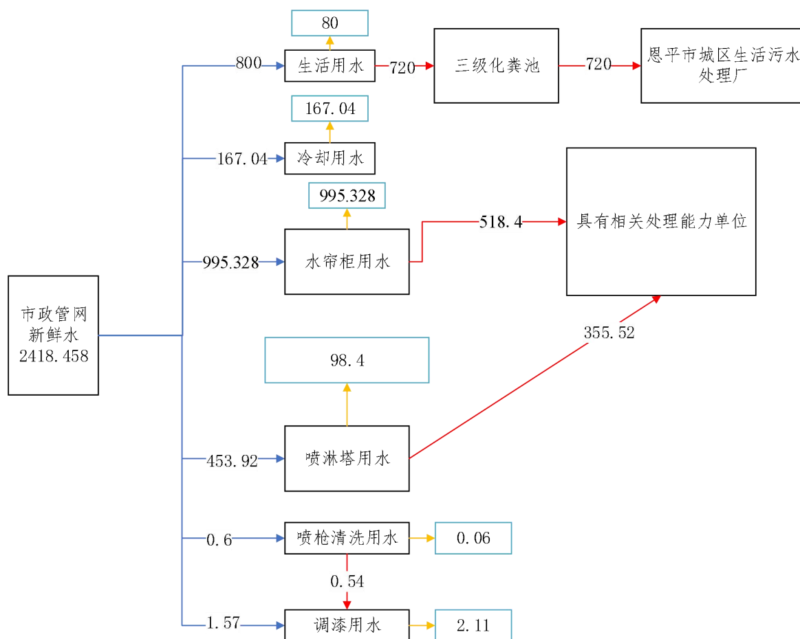
图 1 项目水平衡图 (单位: m³/a)
