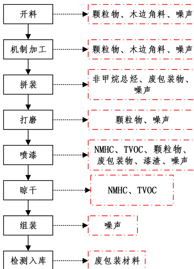
图 6 本项目音响产品生产工艺流程图
