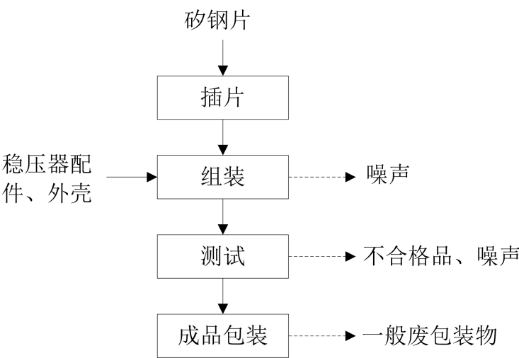
图 2-4 本项目稳压器生产工艺流程及产污环节
