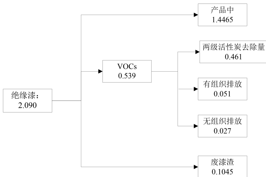
图 2-1 项目含 VOCs 物料平衡图 单位：t/a
