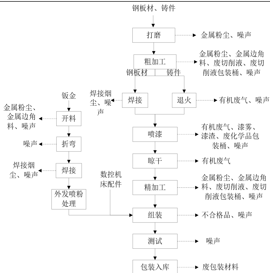
图 2-2 本项目数控机床生产工艺流程及产污环节
