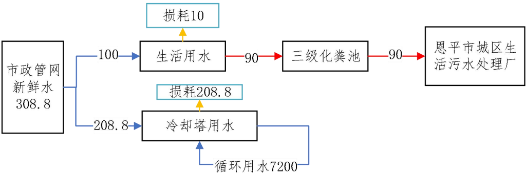
图 2 项目水平衡图 (单位: m³/a)
