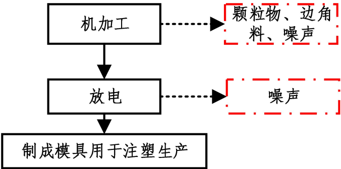
图 2 本项目塑料制品配套模具生产工艺流程及产污过程图
