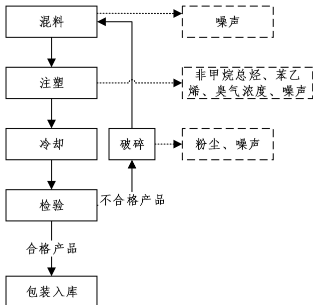
图3 本项目塑料制品生产工艺流程及产污过程图
