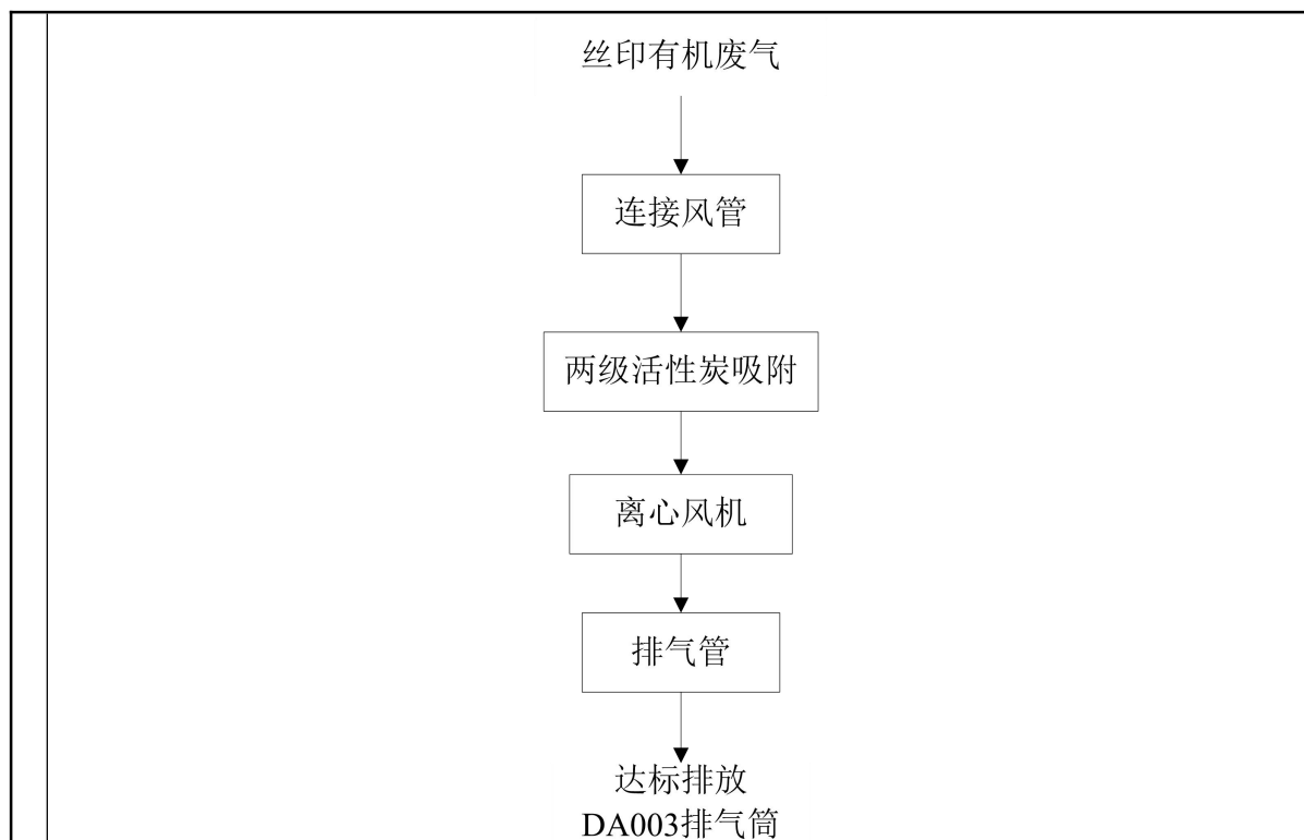
图 4-3 项目丝印有机废气处理工艺流程
