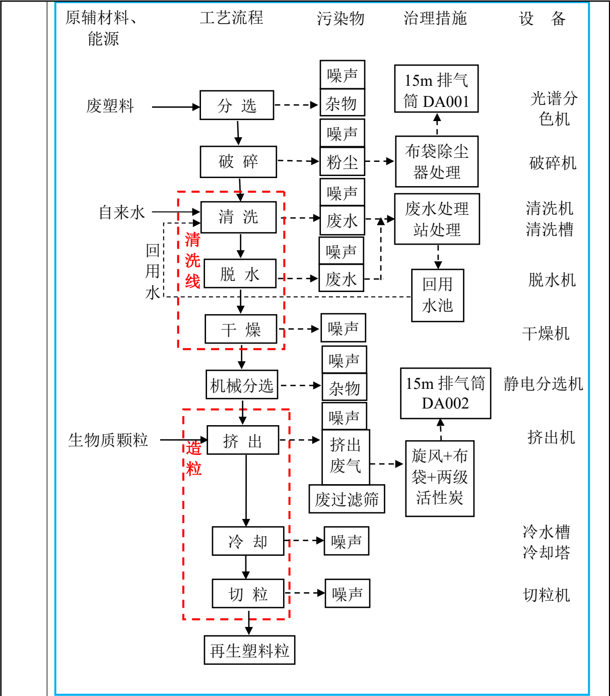
图 2-3 项目再生塑料粒生产工艺流及产污环节
