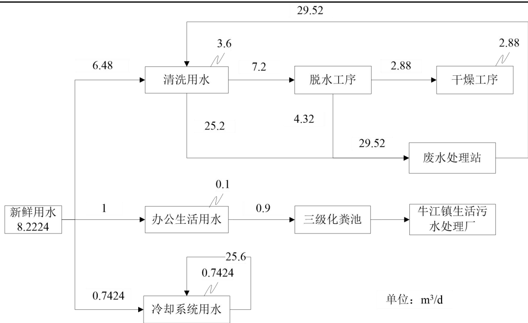
图 2-2 本项目水平衡图
