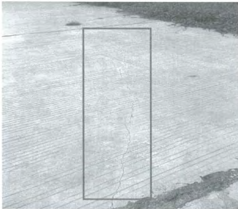
图 26 路面裂缝
