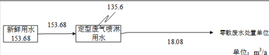
图 2-1 本项目水平衡图
