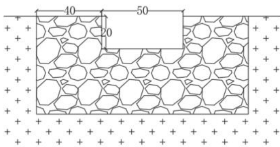
图 4-8 1#、2#、4#、5#、6#截水沟大样图
