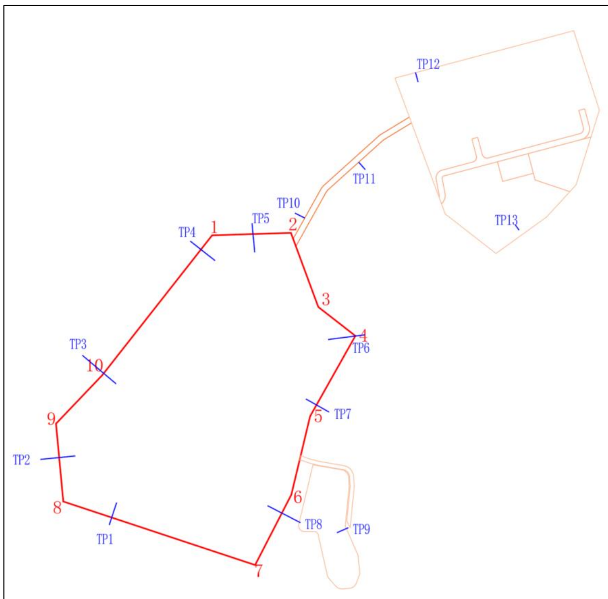
图 3-7 土质边坡位置分布示意图
