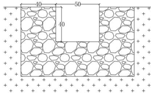
图 4-9 3#截水沟大样图
