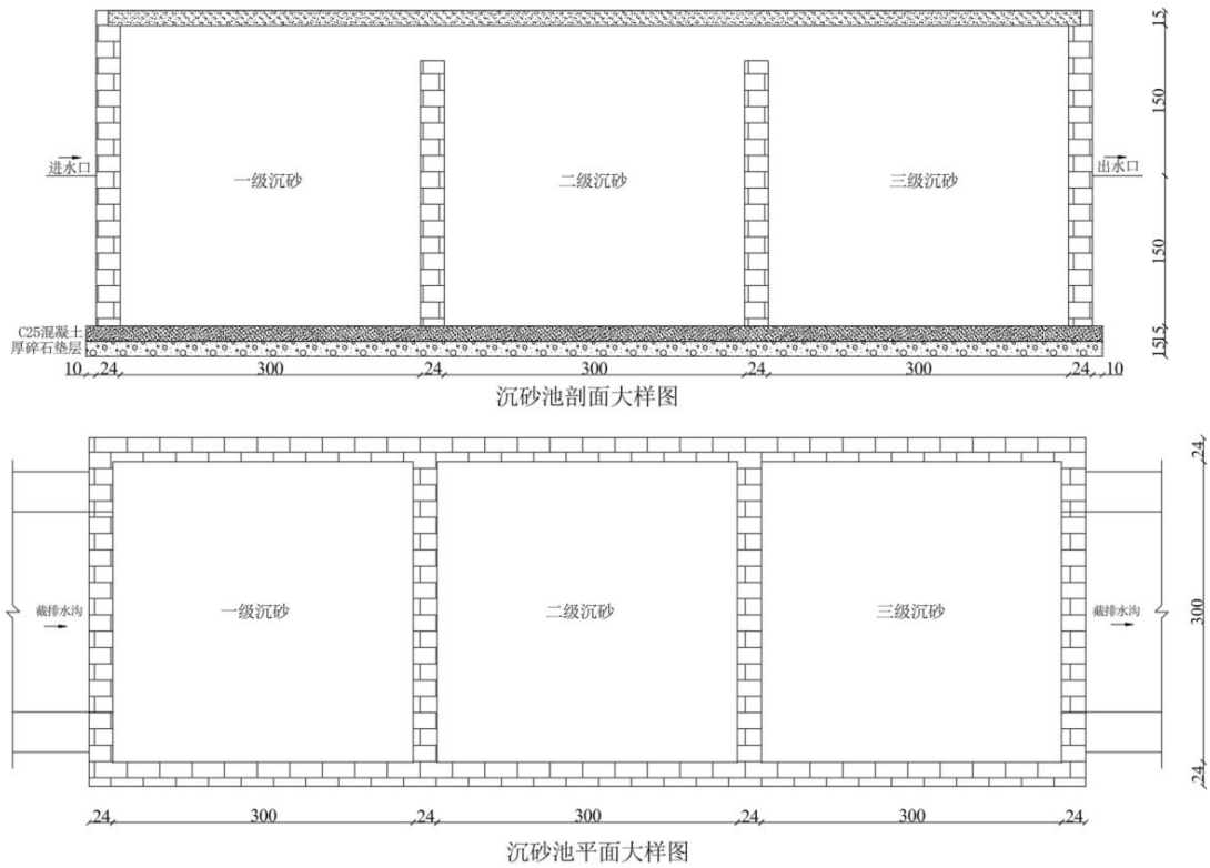
图 4-15 6#沉砂池设计大样图（单位：cm）
