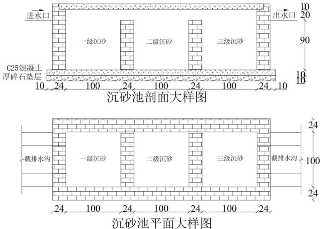
图 4-14 1#、2#、3#、4#、5#、7#、8#沉砂池设计大样图（单位：cm）
