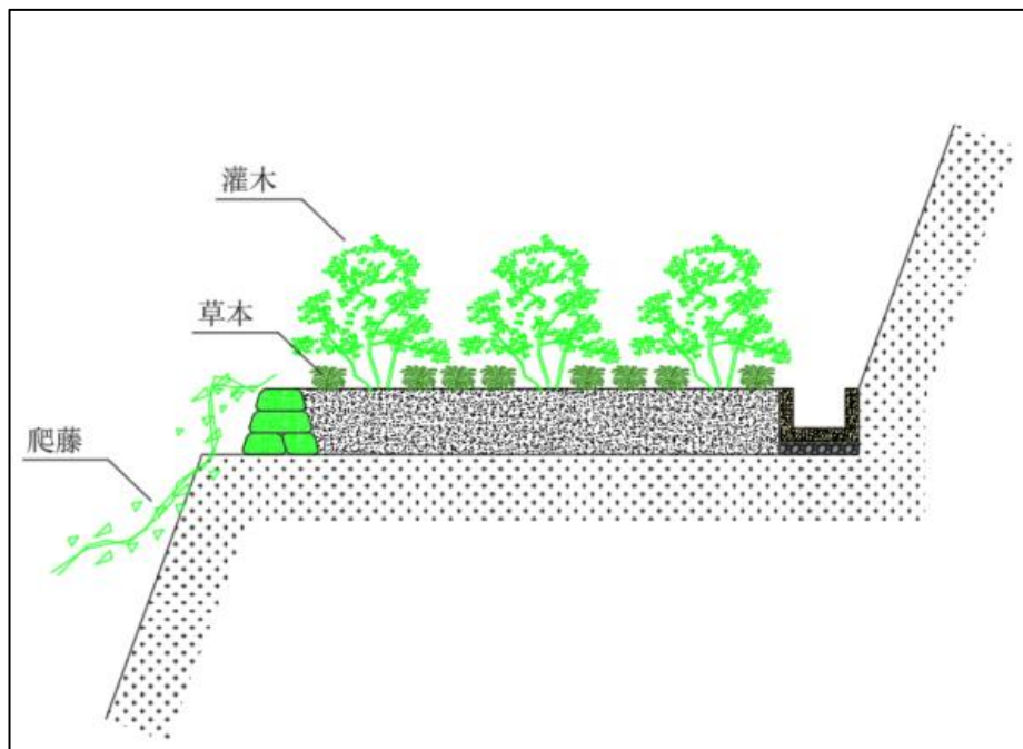
图 4-17 露天采场台阶复垦大样图
