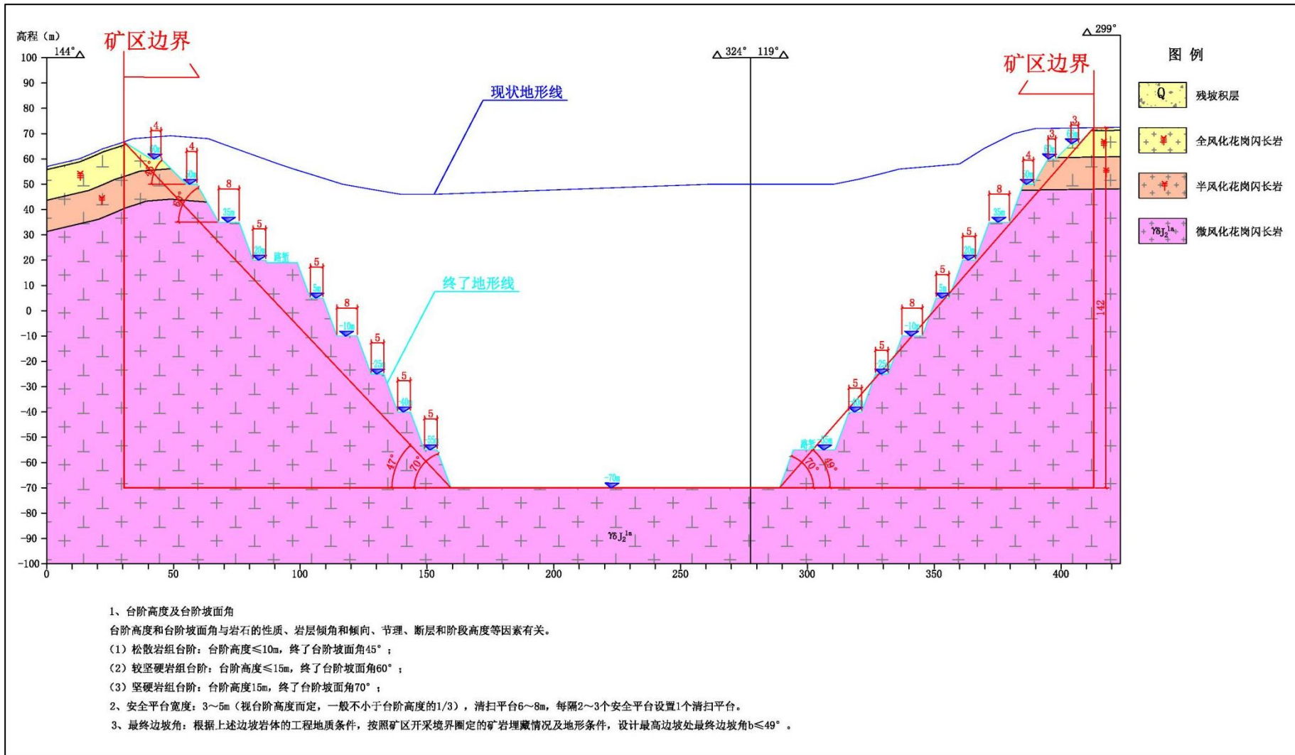
图 1-8 开采终了剖面图（来源于：《开采方案》）
