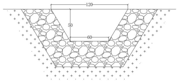
图 4-11 8#截水沟大样图
