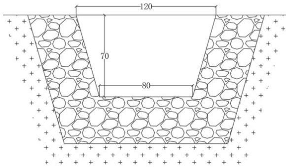
图 4-10 7#截水沟、1#排水沟大样图
