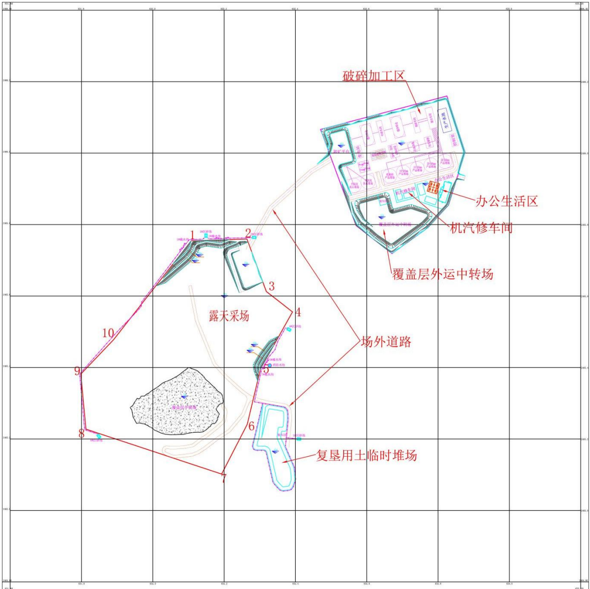
图 1-6 基建总平面布置图（来源于：《开采方案》）
