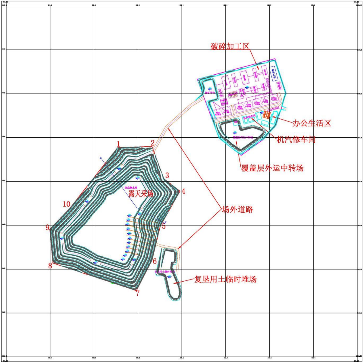
图 1-7 终了总平面布置图（来源于：《开采方案》）
