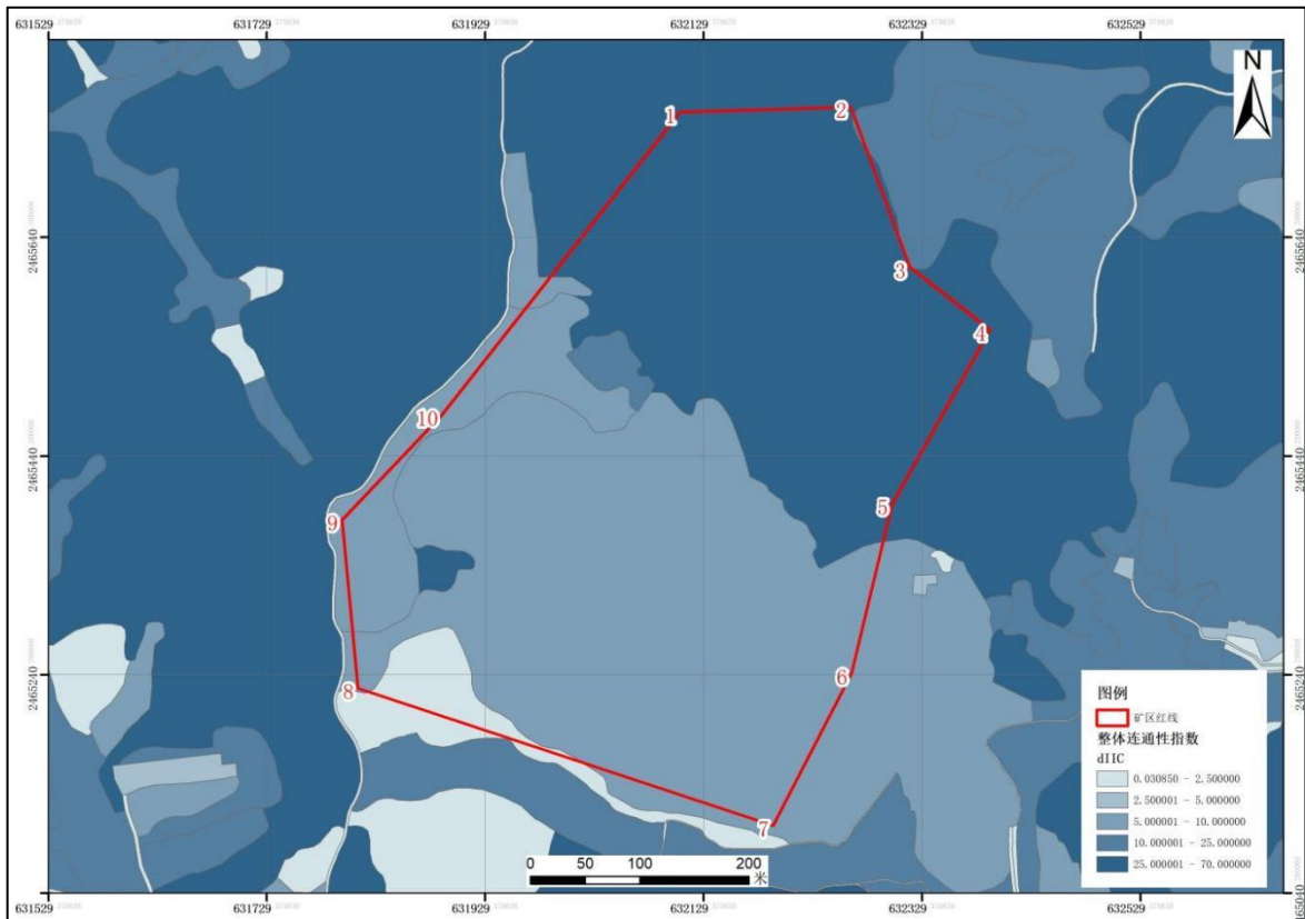
图 2-7 矿区整体连通性指数（IIC）分析结果
