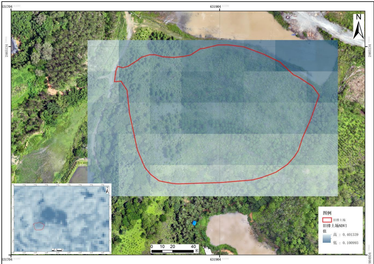
图 3-4 旧排土场 NDVI 图
