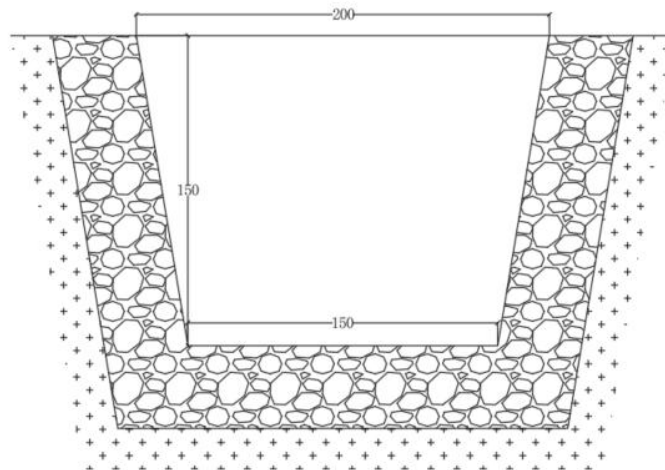
图 4-12 9#截水沟大样图
