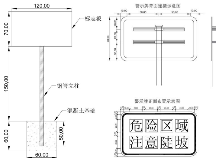
图 4-18 警示牌布置示意图
