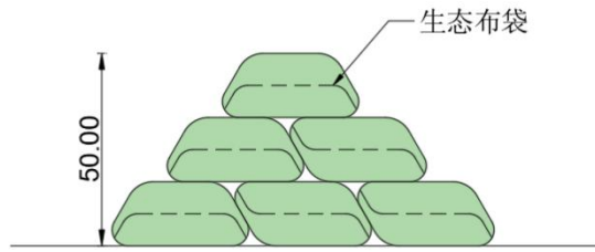
图 4-16 台阶外缘生态布袋挡土墙截面示意图
