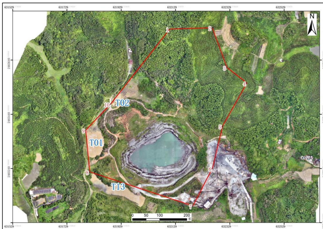
图 2-2 矿区地表水体分布图
