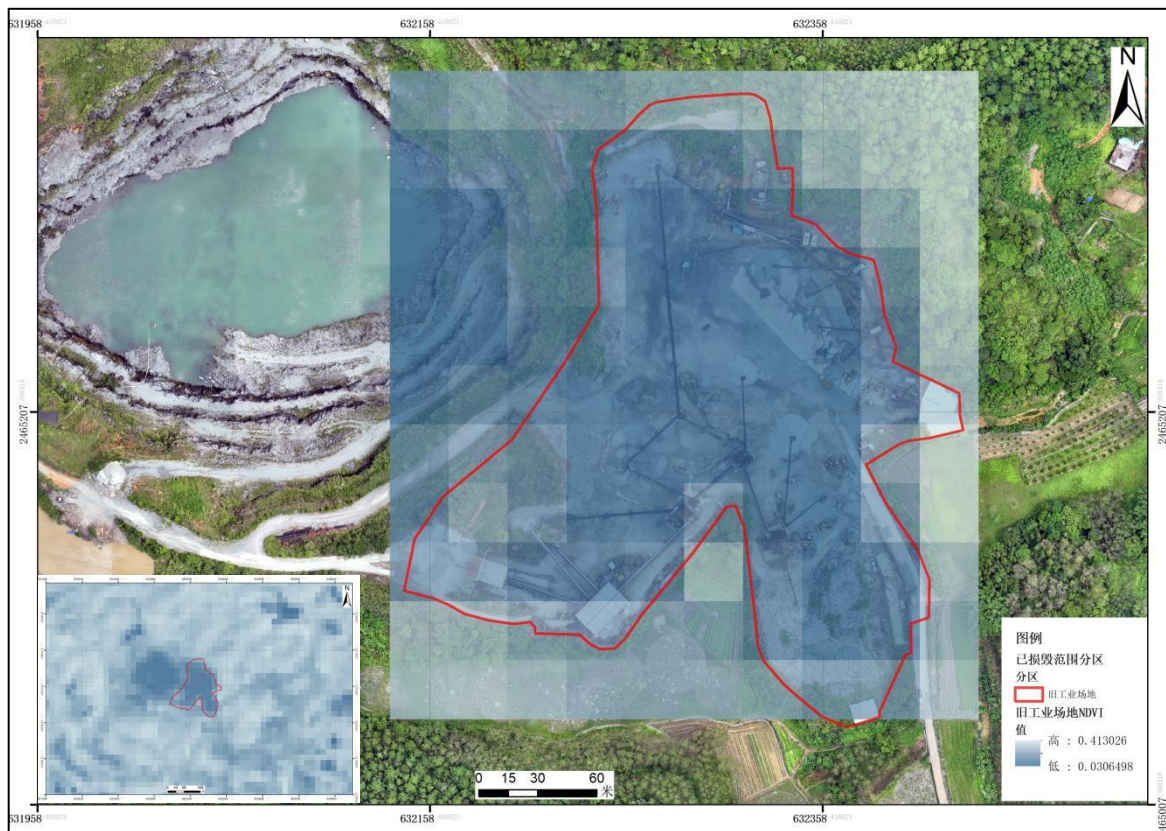
图 3-3 旧工业场地的 NDVI 图
