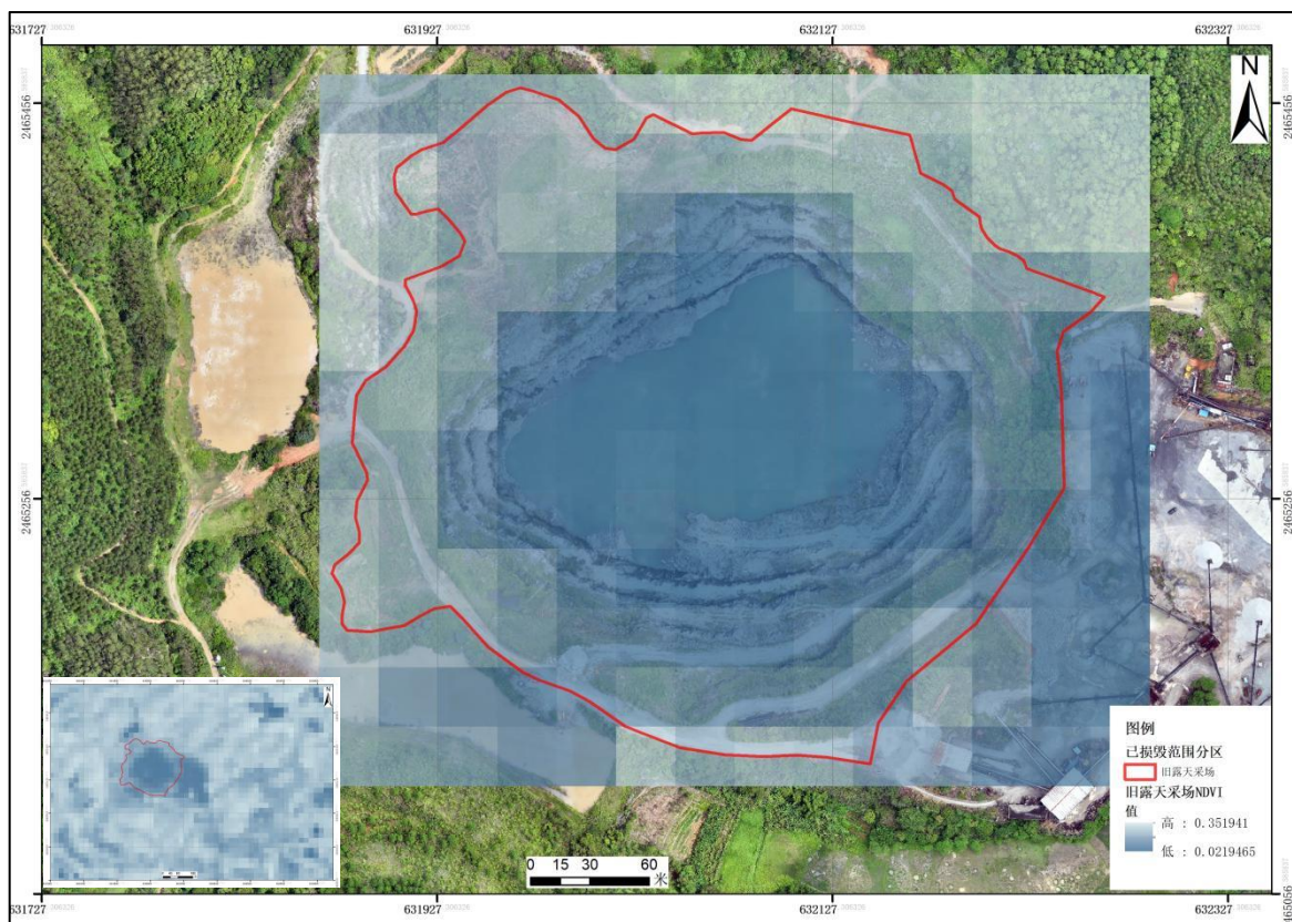
图 3-2 旧露天采场 NDVI 图
