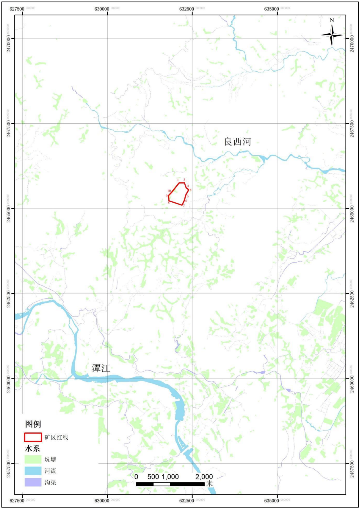
图 2-1 区域地表水体分布图
