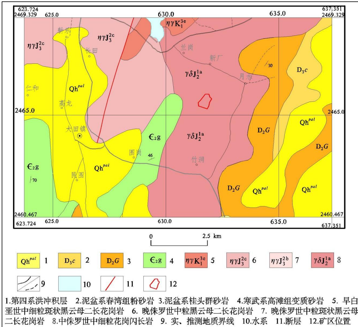
图 2-10 区域地质图 (据 1: 25 万江门市幅)
