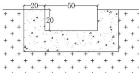
图 4-13 2#排水沟、其他排水沟大样图
