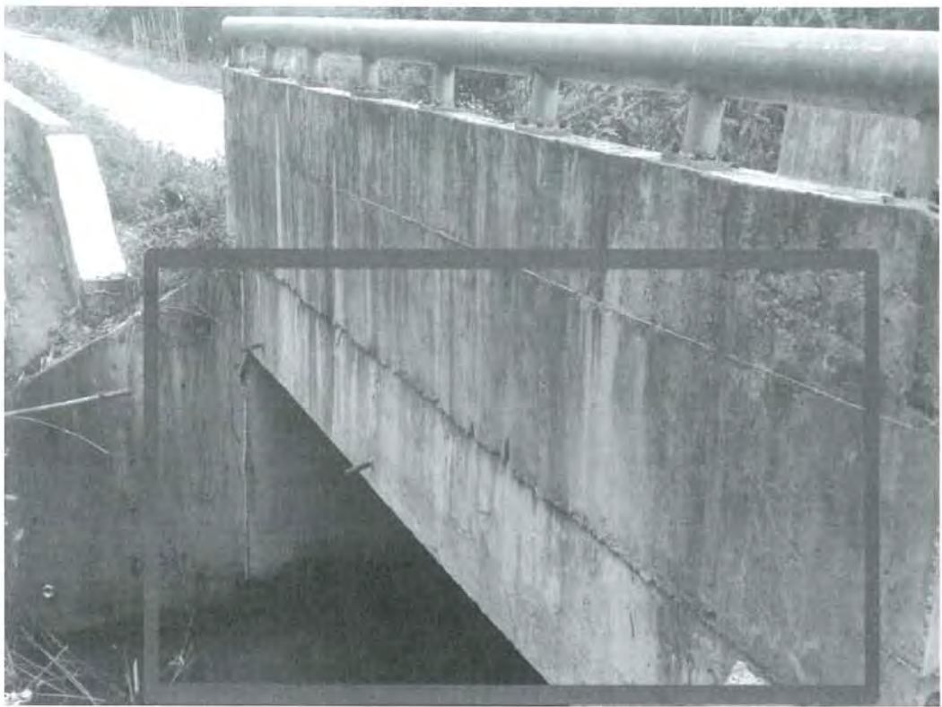
图 7 桥面防撞墙与桥面错位
