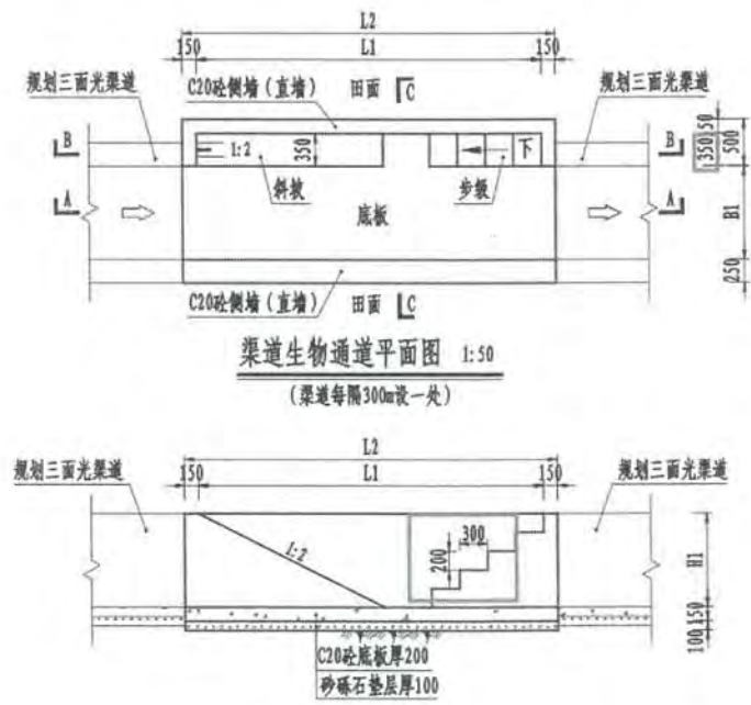
图 14 生物通道设计图
