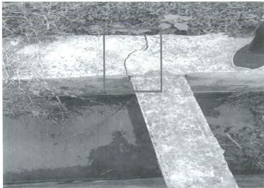
图 10 渠道裂缝及淤积
