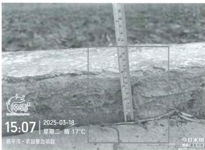
图 19 路面下沉达 90mm
