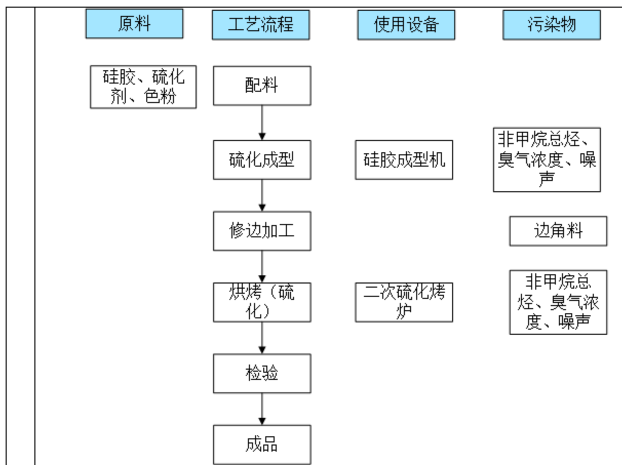
图 2-4 硅胶制品生产工艺流程图
