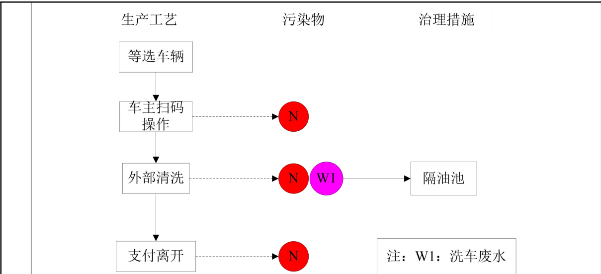
图 2-7 洗车工艺流程图及产污环节
