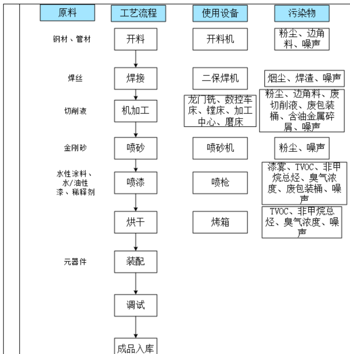
图 2-2 项目数控设备生产工艺流程图
