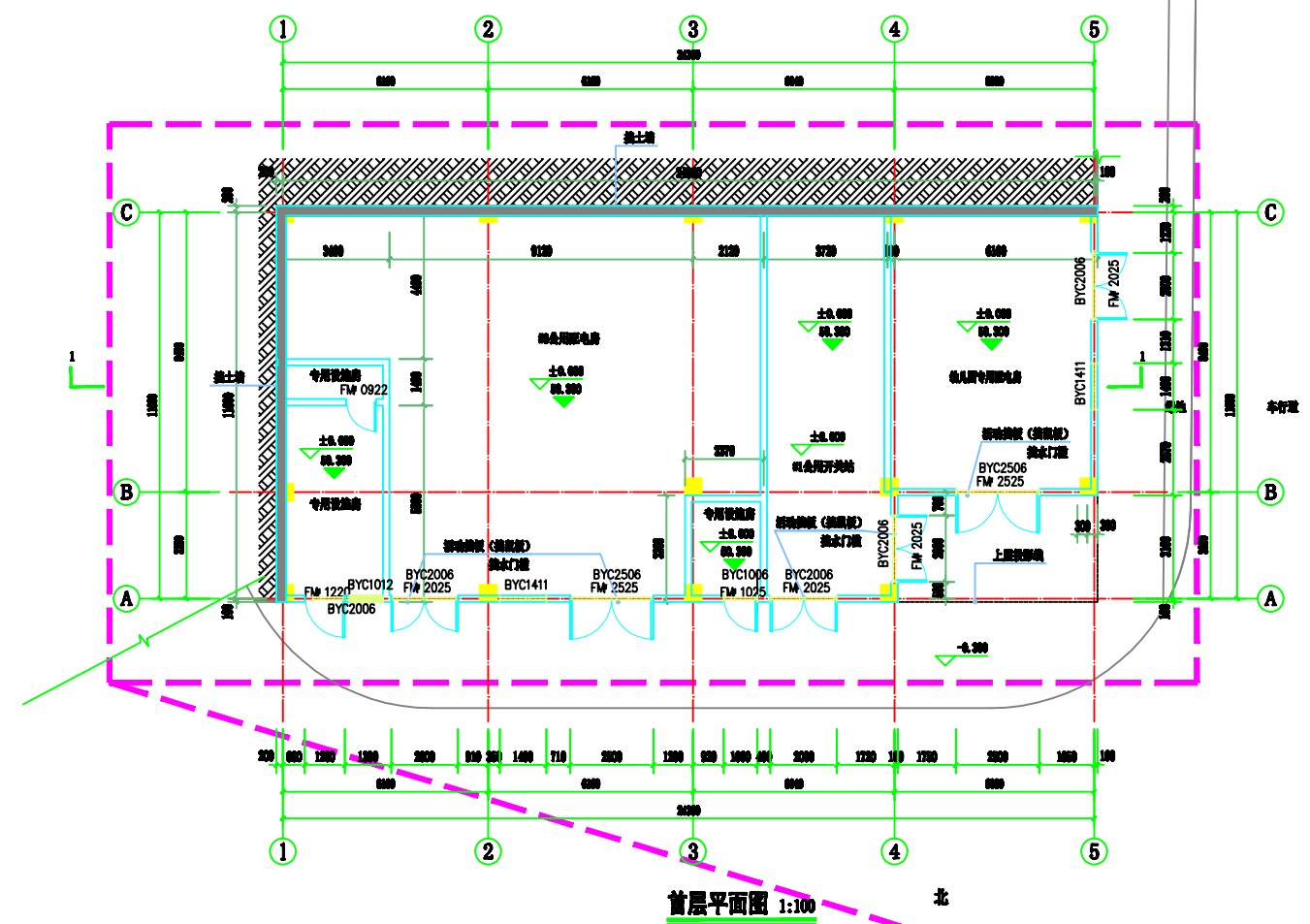
首层平面图 1:100
