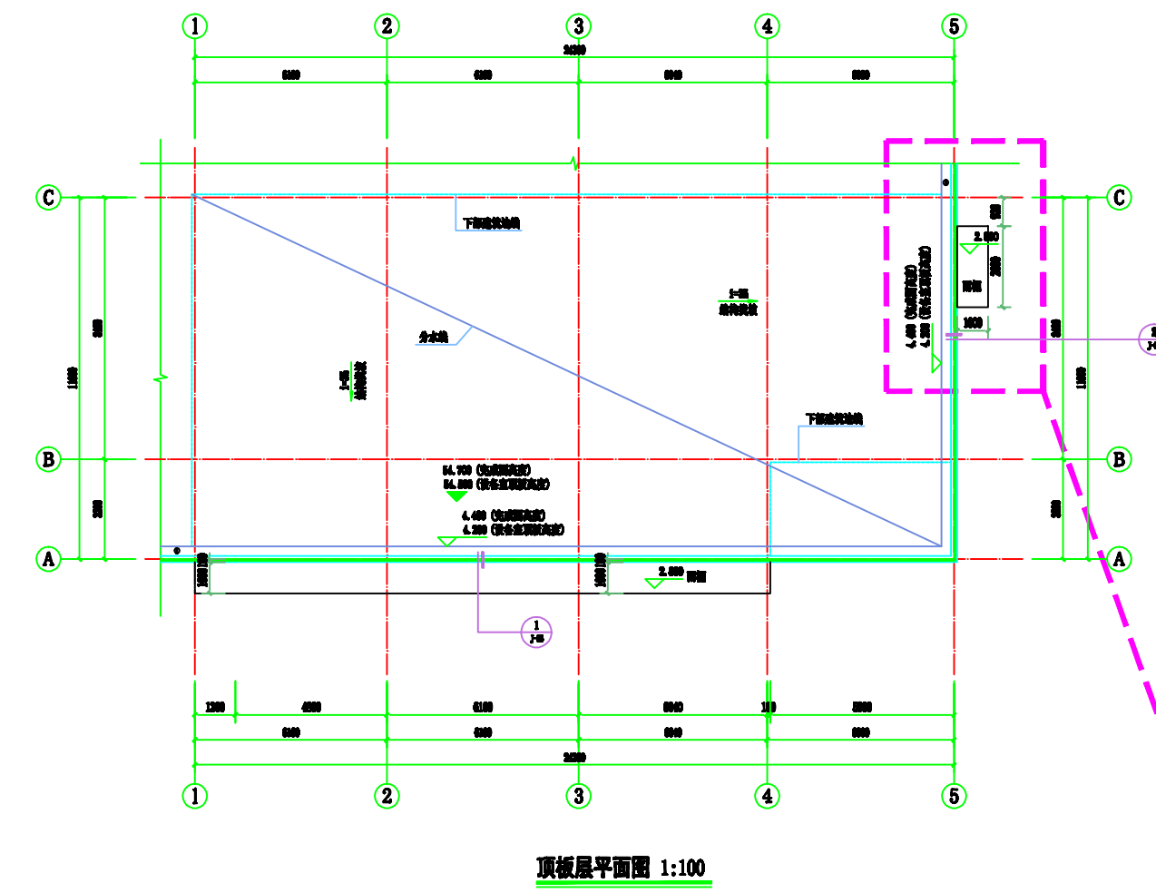
屋顶平面图 1:100
