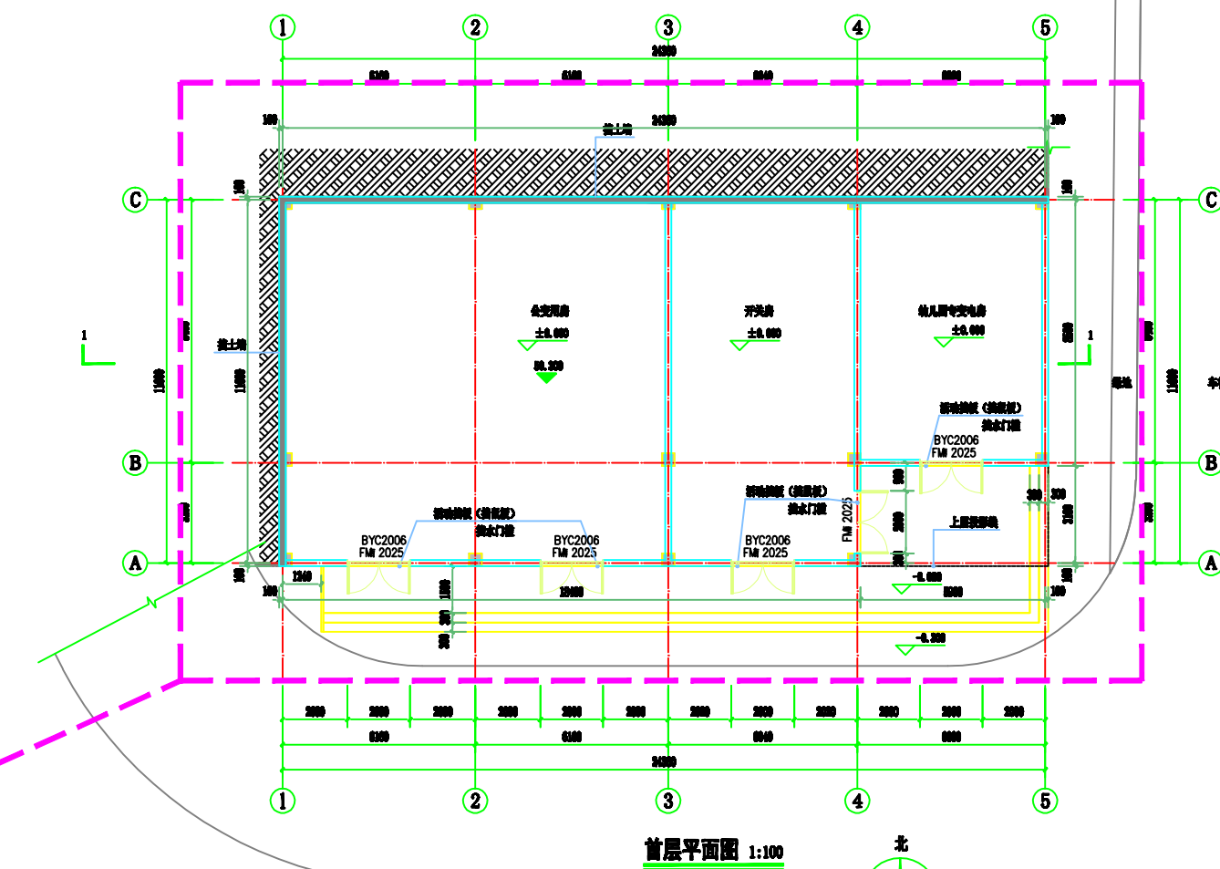
首层平面图 1:100
