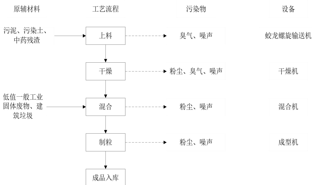
图 2-2 节能新型燃料棒生产工艺流程及产污环节图
