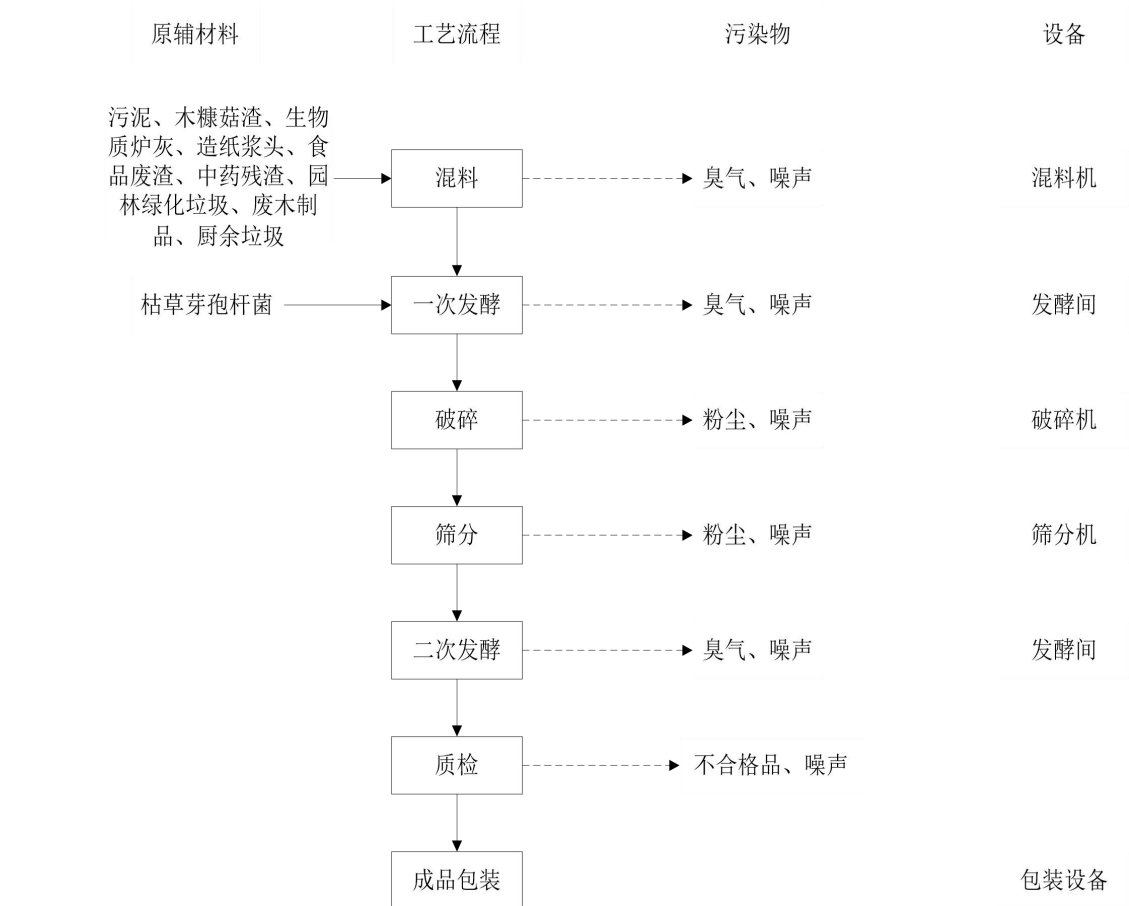
图 2-3 营养土生产工艺流程及产污环节图
