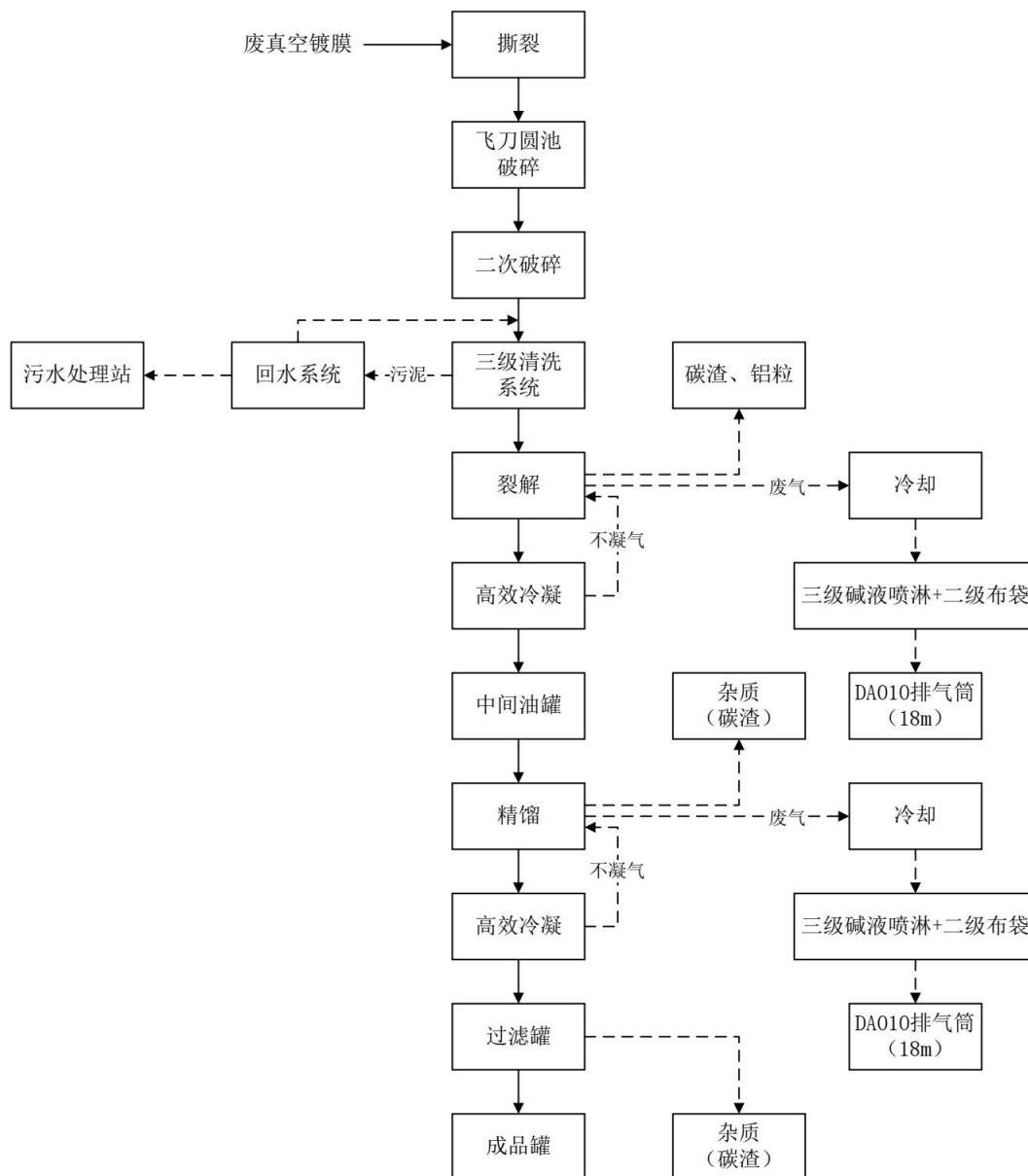
图 2-11 废真空镀膜处理工艺流程及产污节点图
