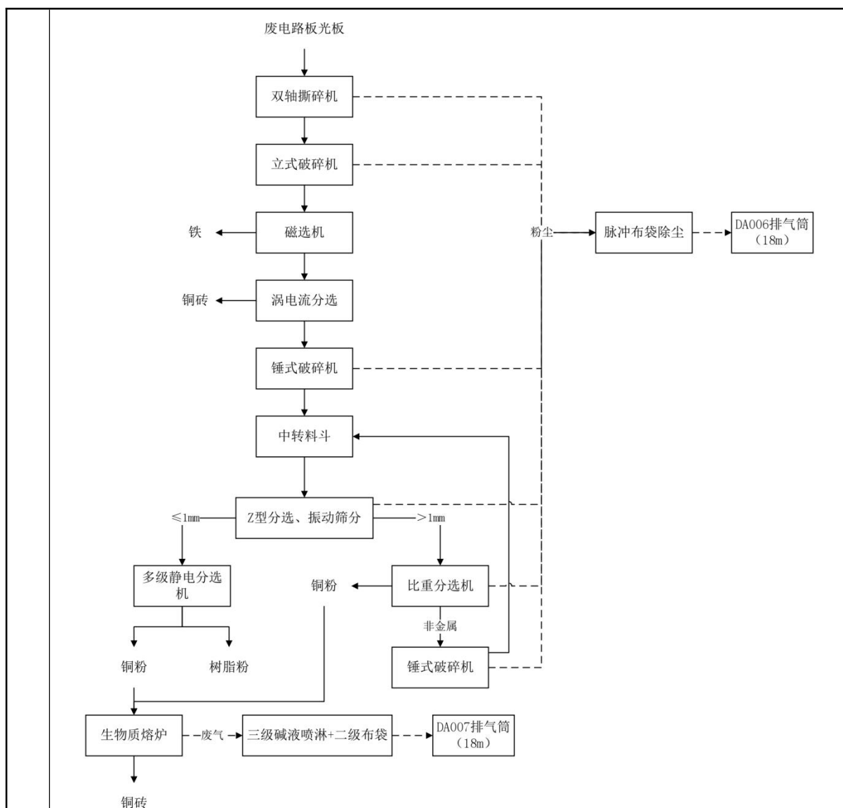
图 2-9 2#废电路板破碎分选处理生产线工艺流程及产污环节图
