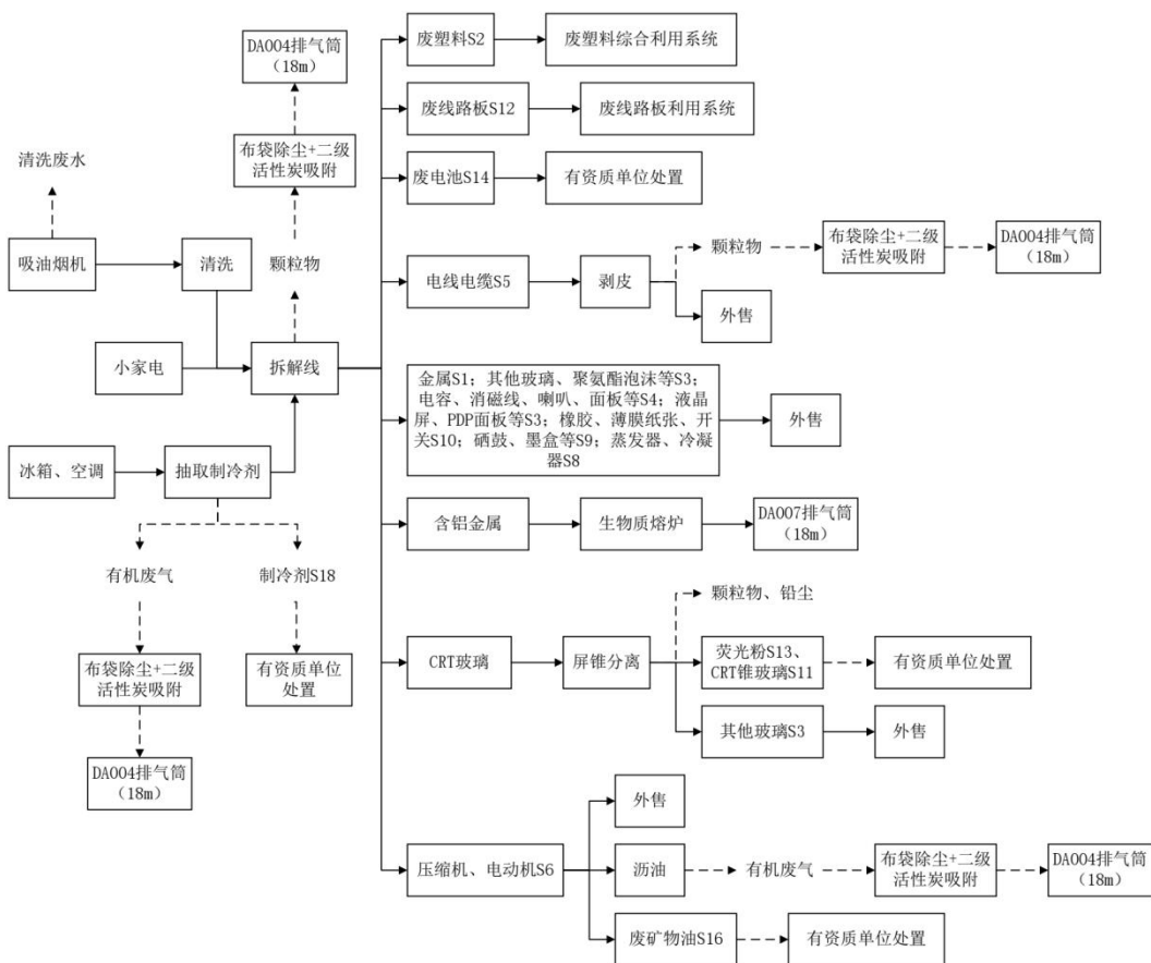
图 2-6 小家电拆解工艺流程及产污环节示意图
