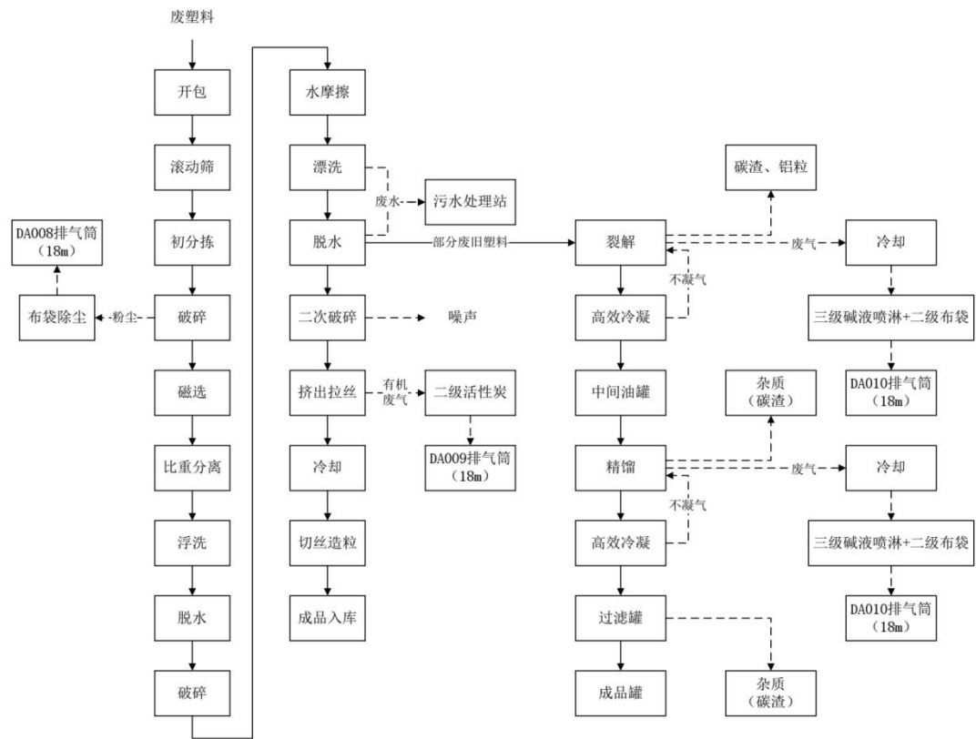
图 2-10 塑料粒及裂解油生产工艺流程及产污节点图
