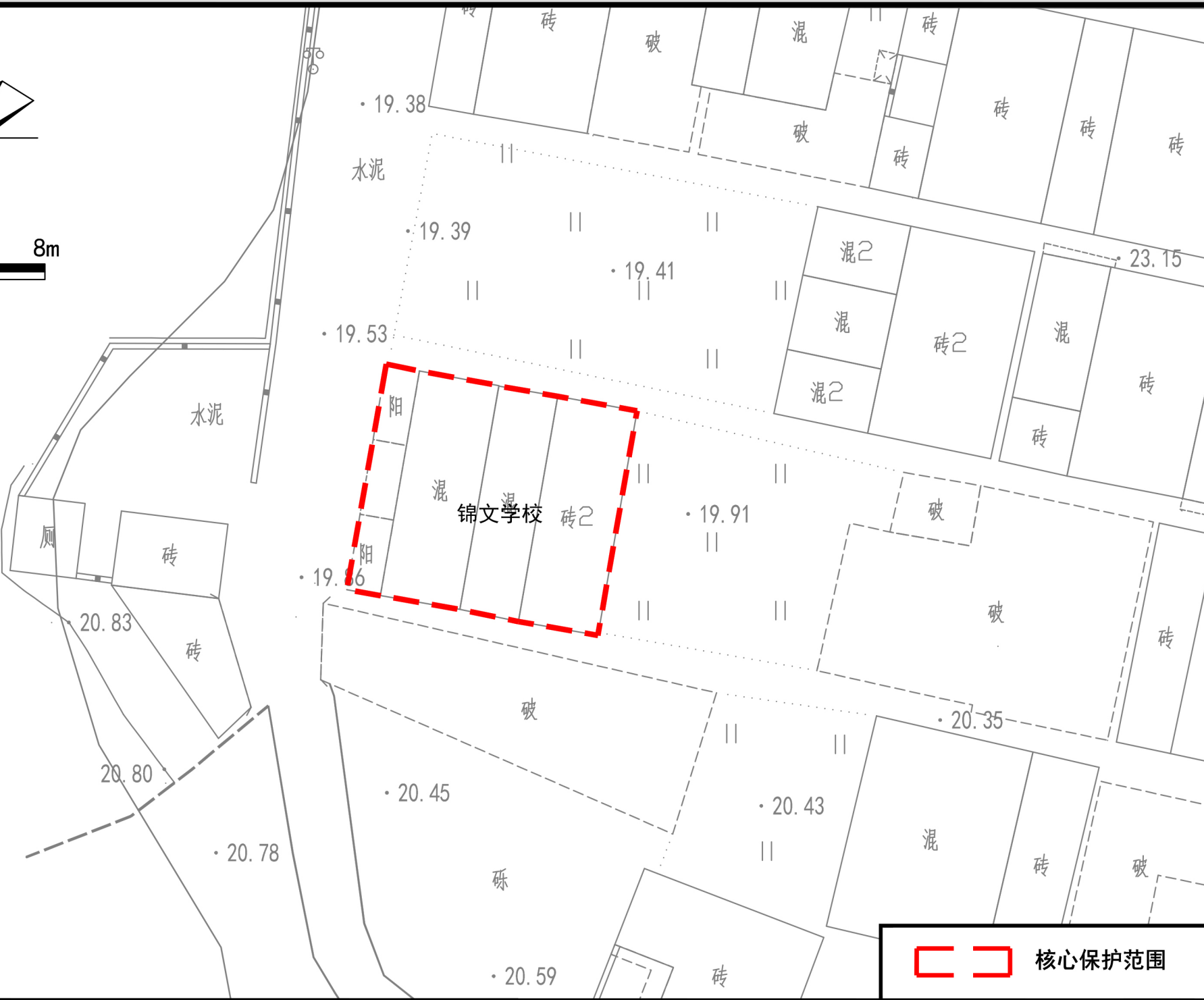
保护范围图
