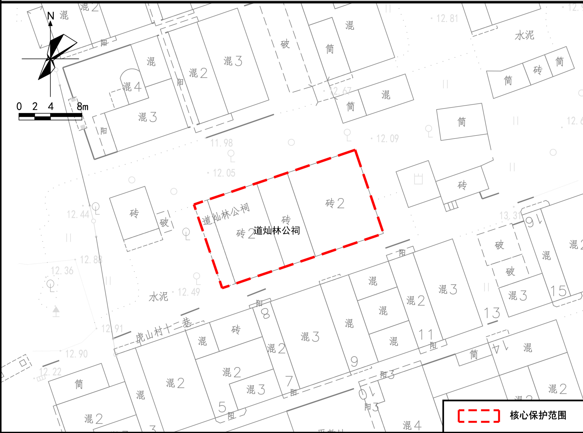
保护范围图
