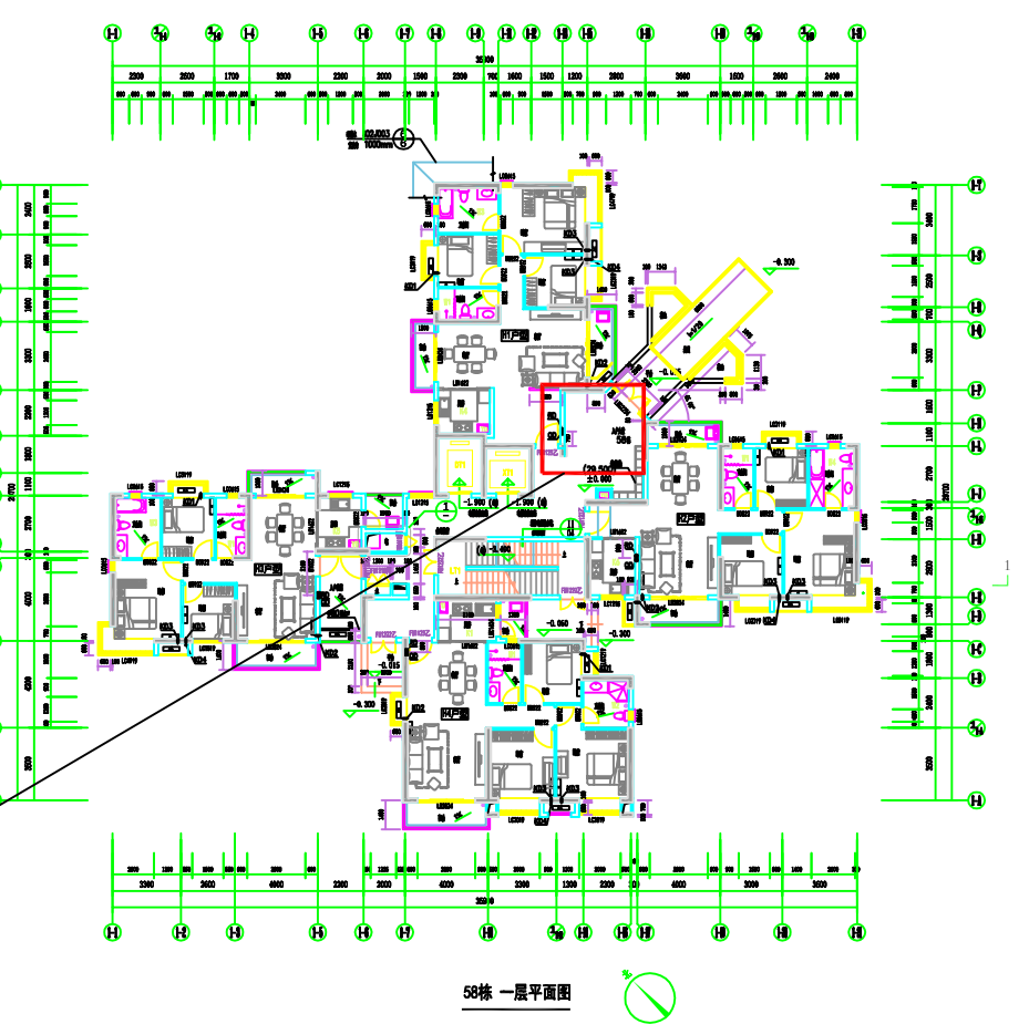
58栋一层（2013年报建方案）
