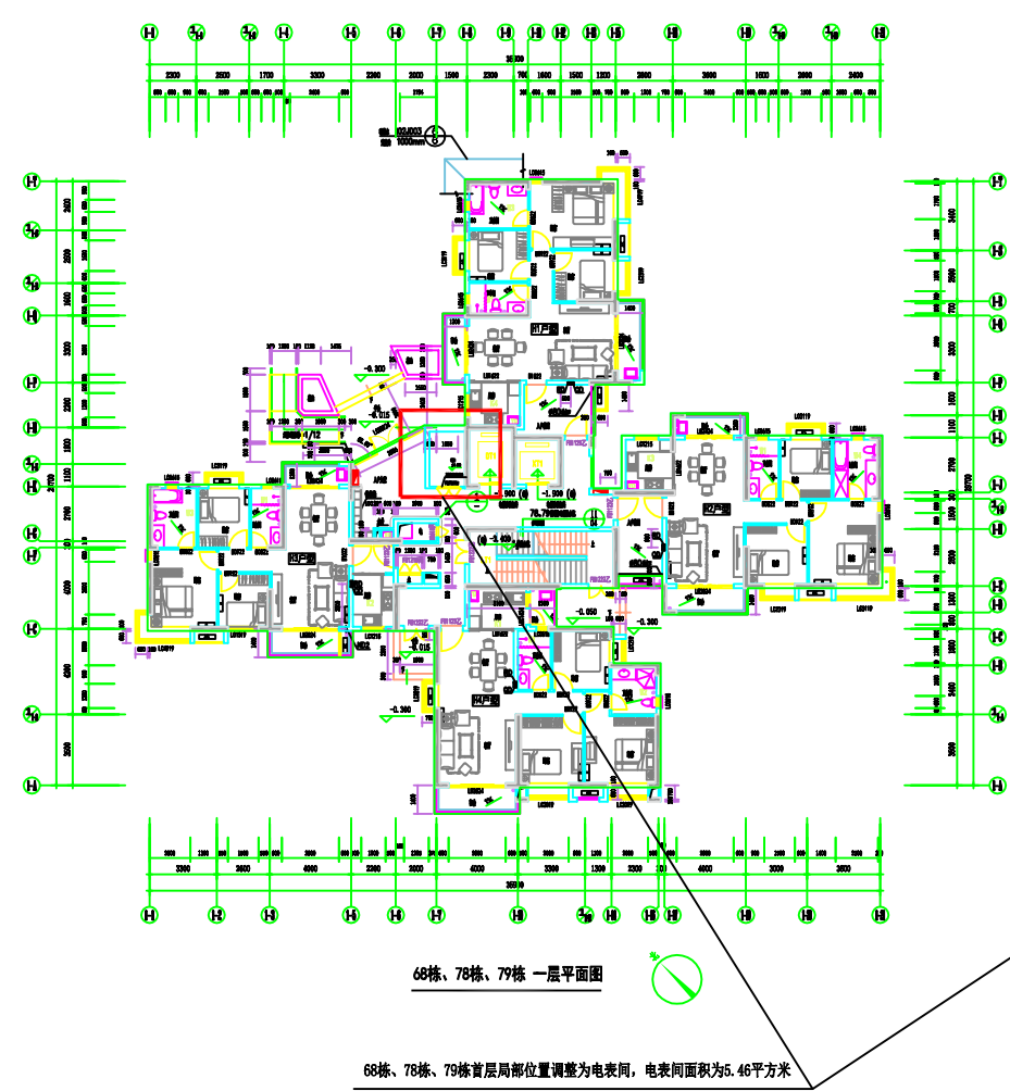
68栋、78栋、79栋一层调整方案
