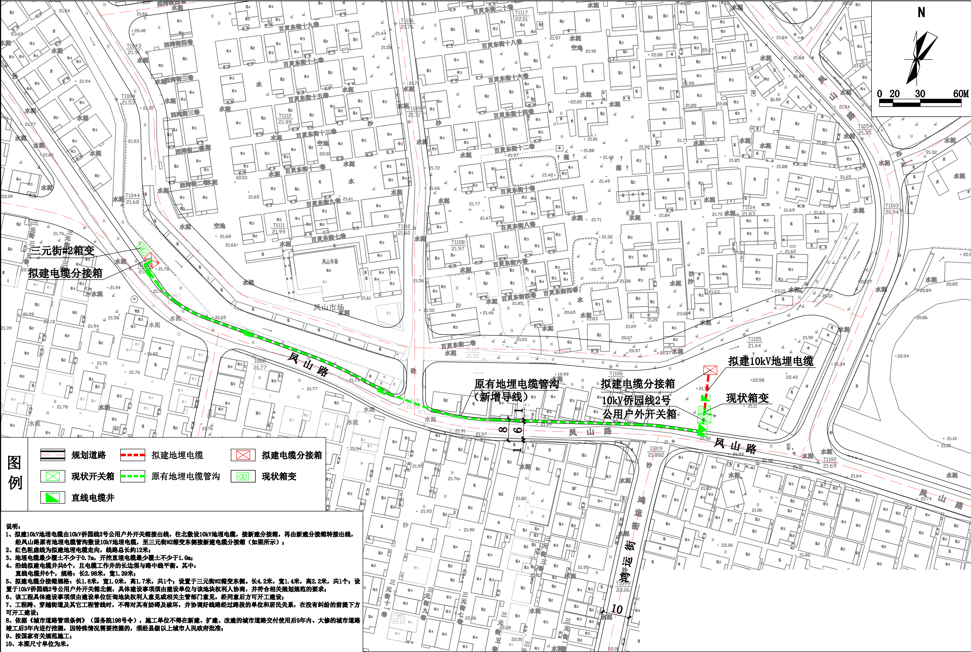
恩平供电局10kV侨园线网架完善工程走向示意图（三）
