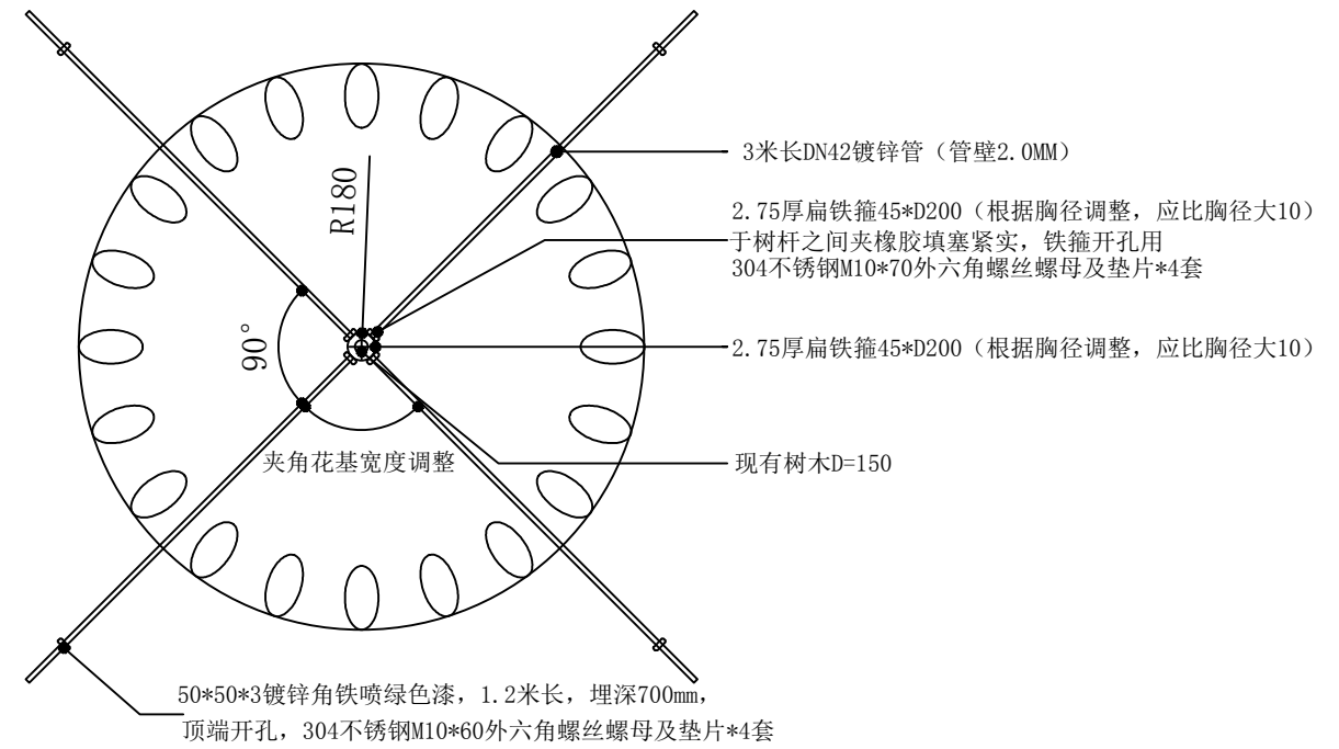
镀锌管支撑平面图 1:40
